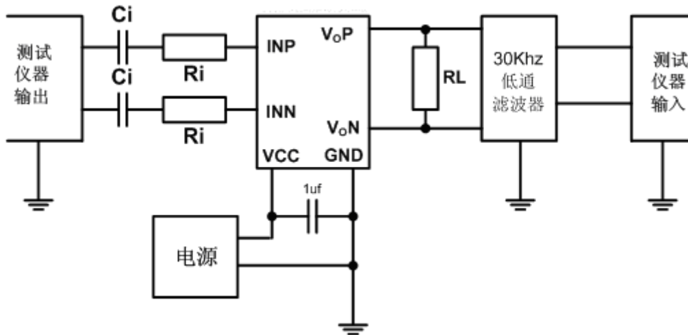
XPT8871 测试连接示意图
