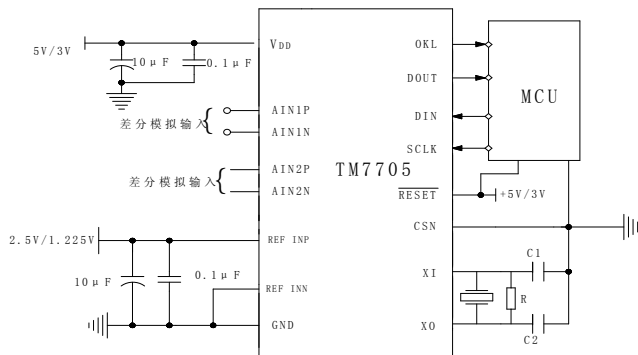
图 5 TM7705 的电路图
